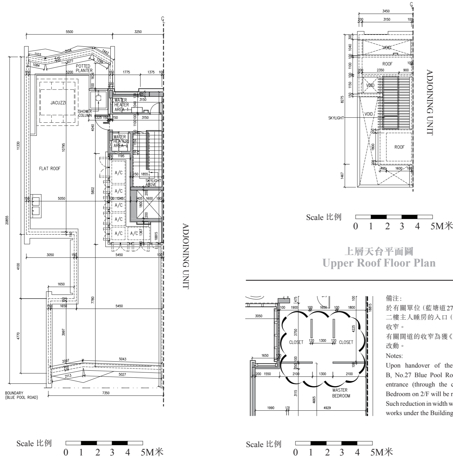
天台平面圖 Roof Floor Plan
