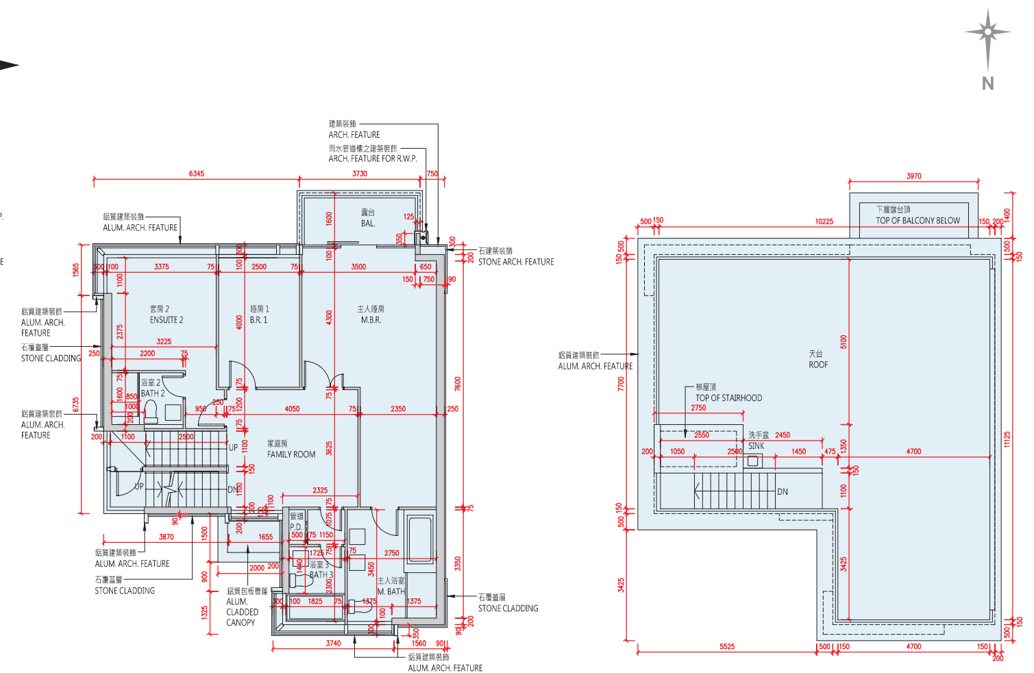
1/F Floor Plan 1樓平面圖
