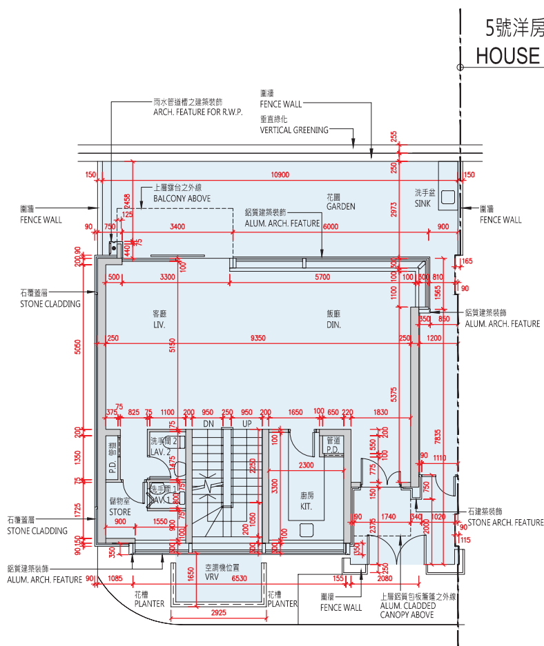
G/F Floor Plan 地下平面圖
