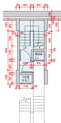
B1/F Floor Plan 地庫1樓平面圖
