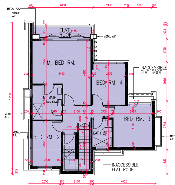
1/F FLOOR PLAN 1樓樓面平面圖
