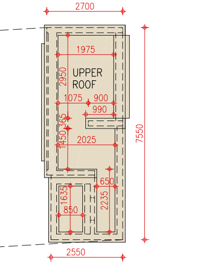
HOUSE LEVEL 3 PLAN 獨立屋第三層平面圖
