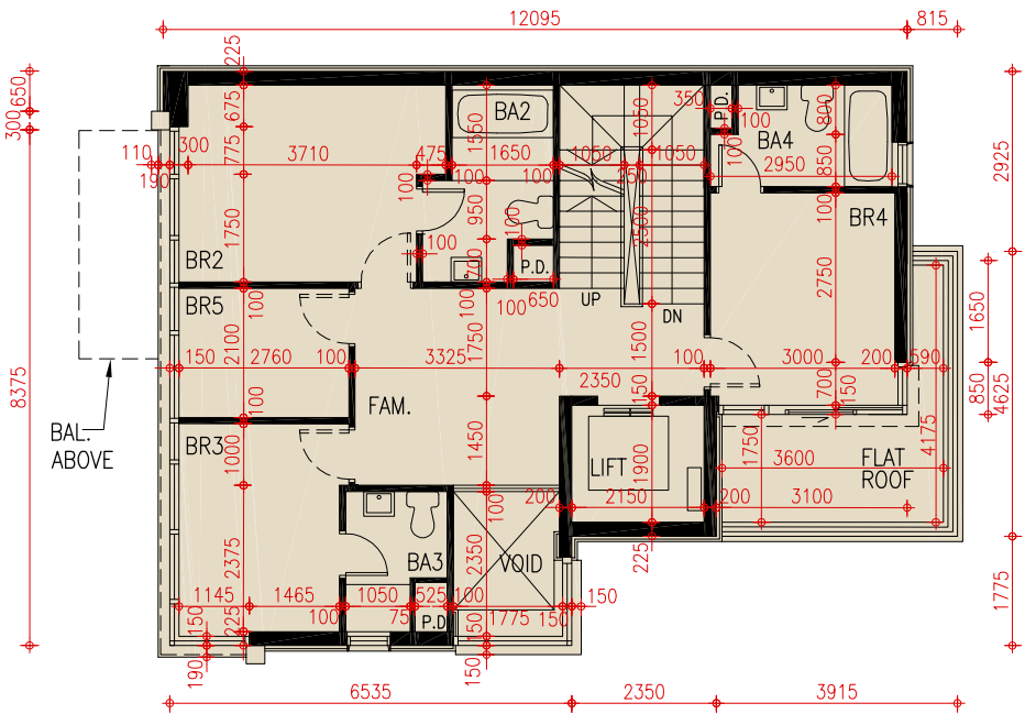
HOUSE LEVEL 2 PLAN 獨立屋第二層平面圖
