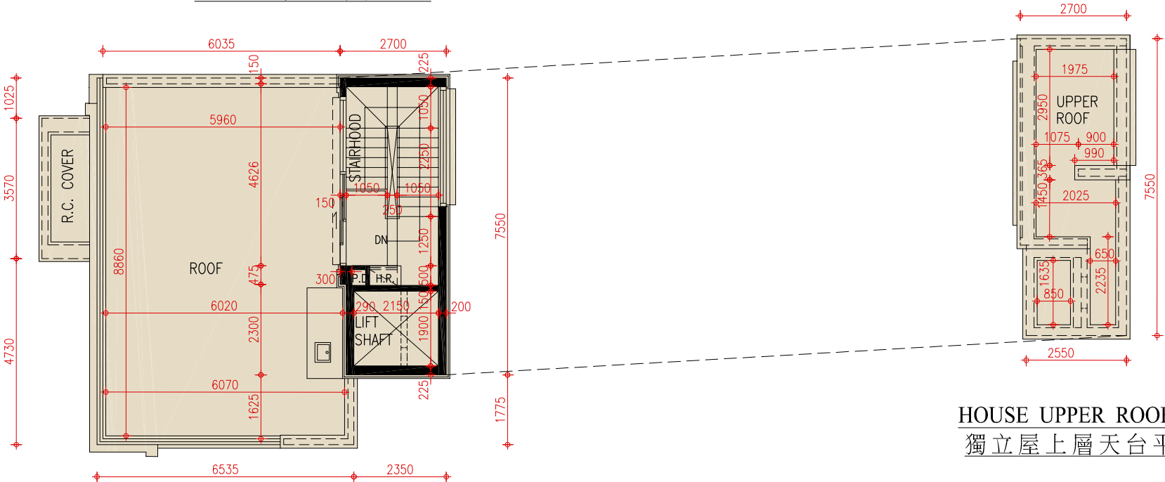
HOUSE ROOF PLAN 獨立屋天台平面圖
