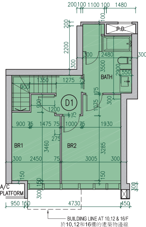
Upper Duplex of Unit D1 (9/F, 11/F, 15/F) 複式單位 D1 上層 (9樓, 11樓, 15樓)
