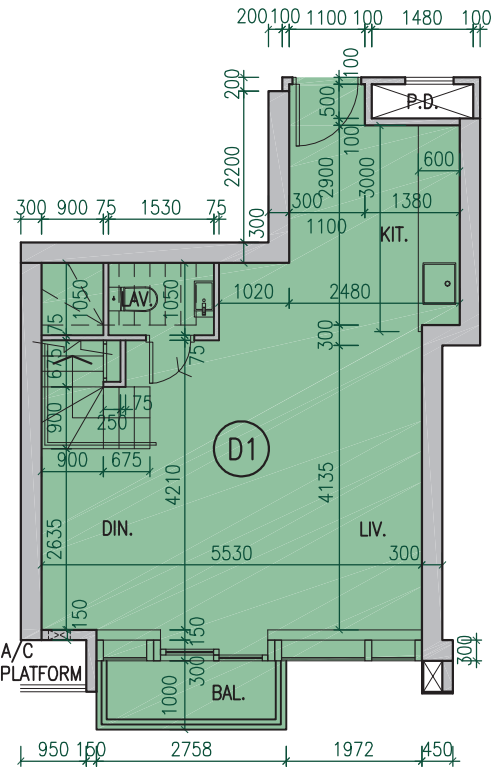
Lower Duplex of Unit D1 (8/F, 10/F, 12/F) 複式單位 D1 下層 (8樓, 10樓, 12樓)
