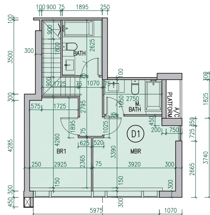
Upper Duplex of Unit D1 (18/F, 20/F, 22/F, 25/F) 複式單位D1上層 (18樓, 20樓, 22樓, 25樓)
