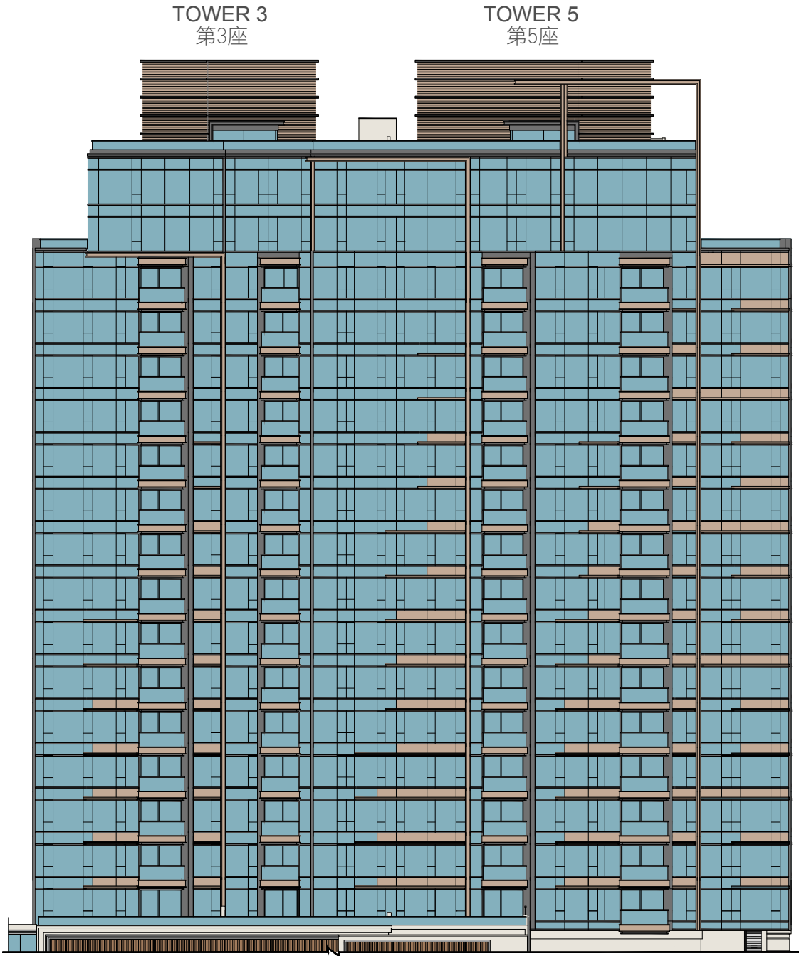
ELEVATION E 立面圖 E
