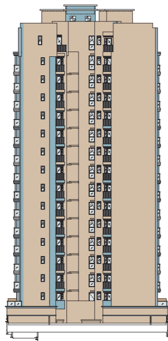
Elevation 1 立面圖 1
