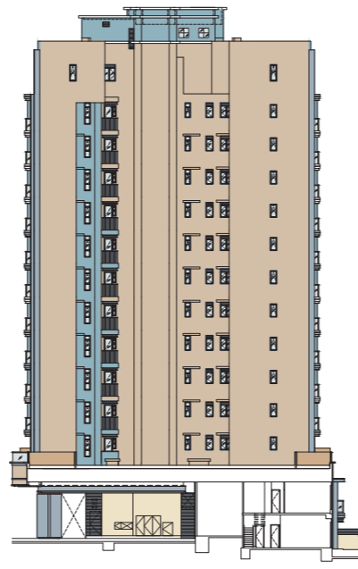
Elevation 2 立面圖 2
