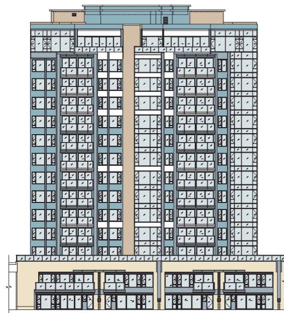
Elevation 1 立面圖 1
