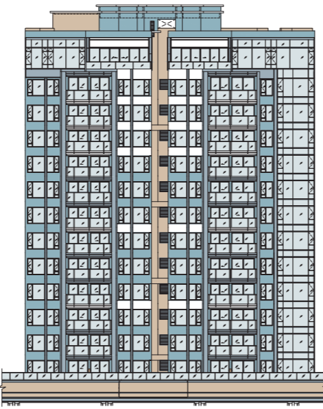
Elevation 4 立面圖 4
