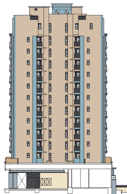
Elevation 2 立面圖 2
