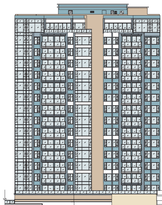
Elevation 4 立面圖 4
