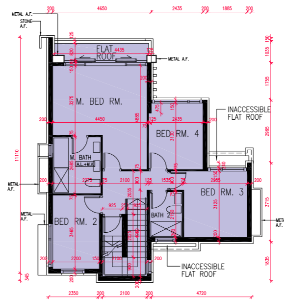
1/F FLOOR PLAN 1樓樓面平面圖
