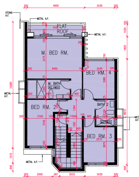
1/F FLOOR PLAN 1樓樓面平面圖
