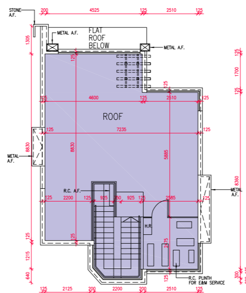
ROOF FLOOR PLAN 天台樓面平面圖
