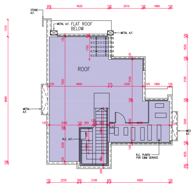
ROOF FLOOR PLAN 天台樓面平面圖
