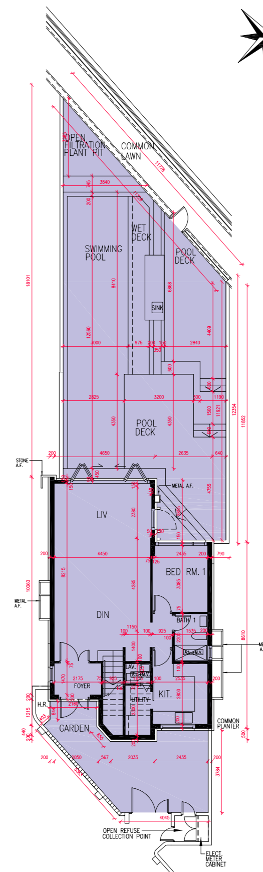
G/F FLOOR PLAN 地下樓面平面圖
