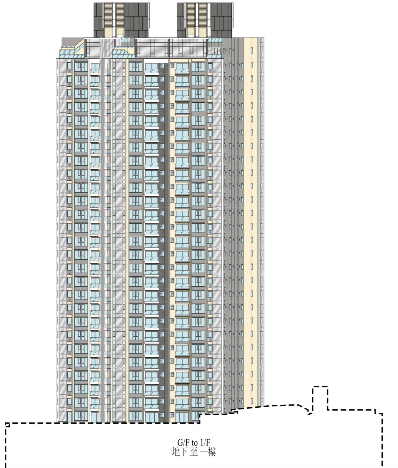
ELEVATION PLAN IV 立面圖 IV
