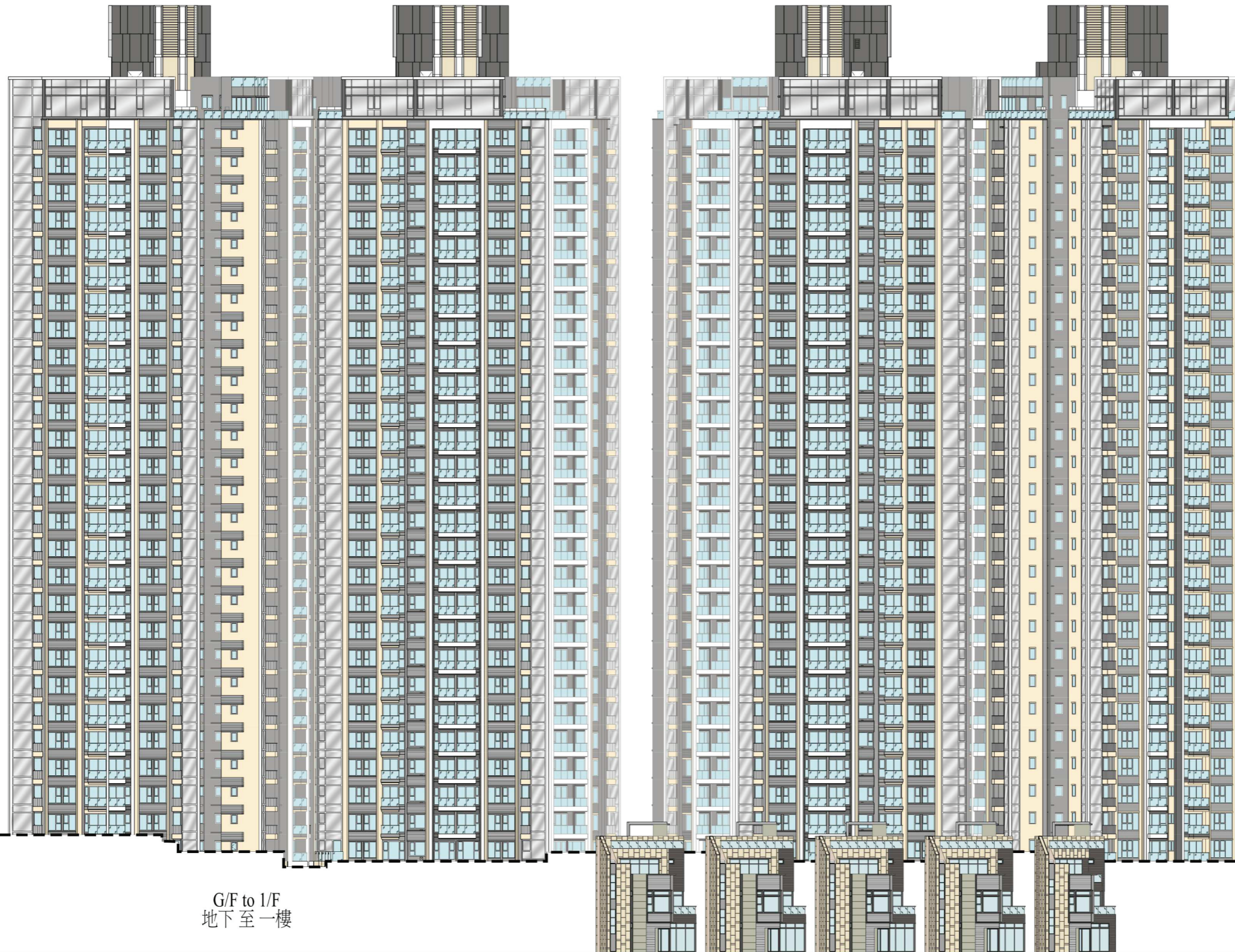
ELEVATION PLAN III 立面圖 III
