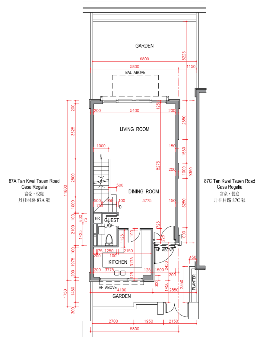
G/F Plan 地面層平面圖
