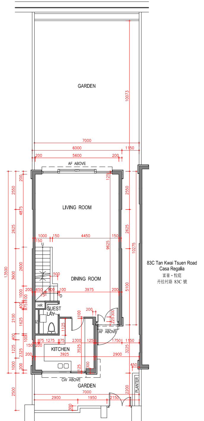
G/F Plan 地面層平面圖
