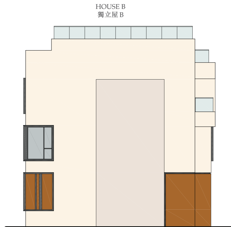
Elevation 10 立面圖 10
