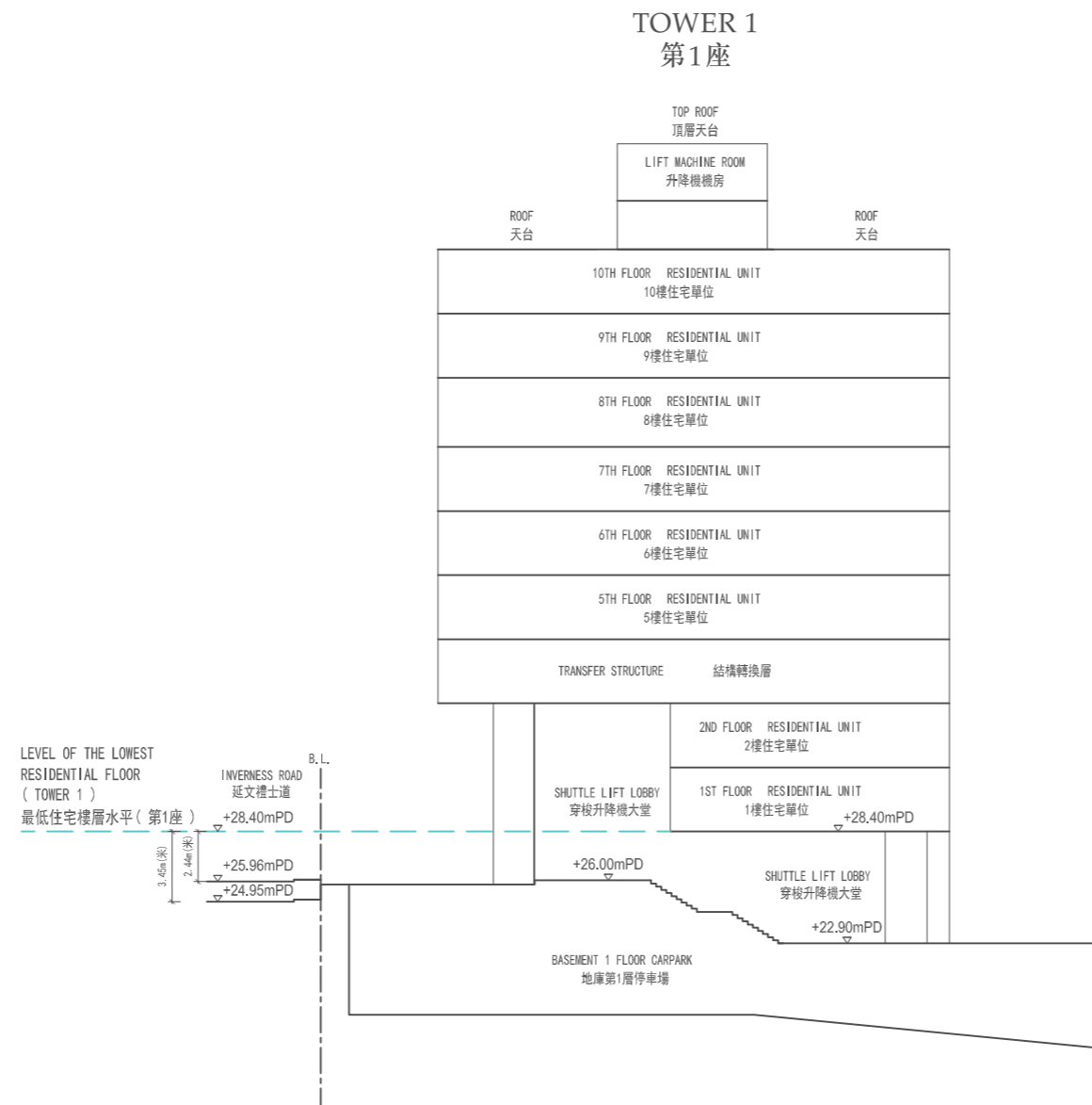
Cross Section Plan A-A 橫截面圖 A-A
