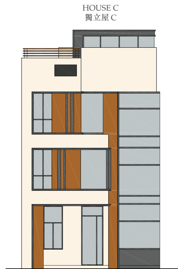
Elevation 15 立面圖 15
