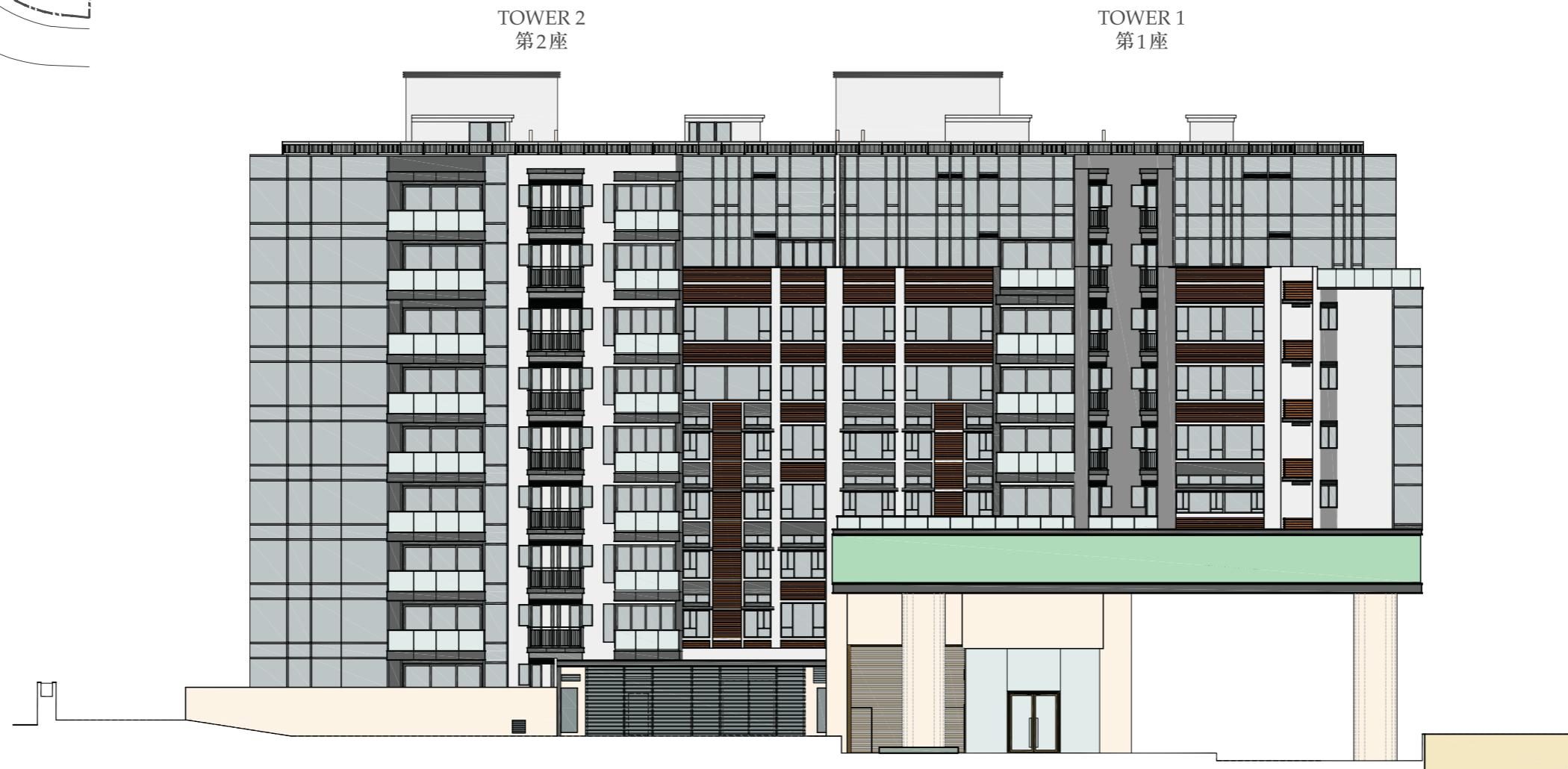
Elevation 1 立面圖 1
