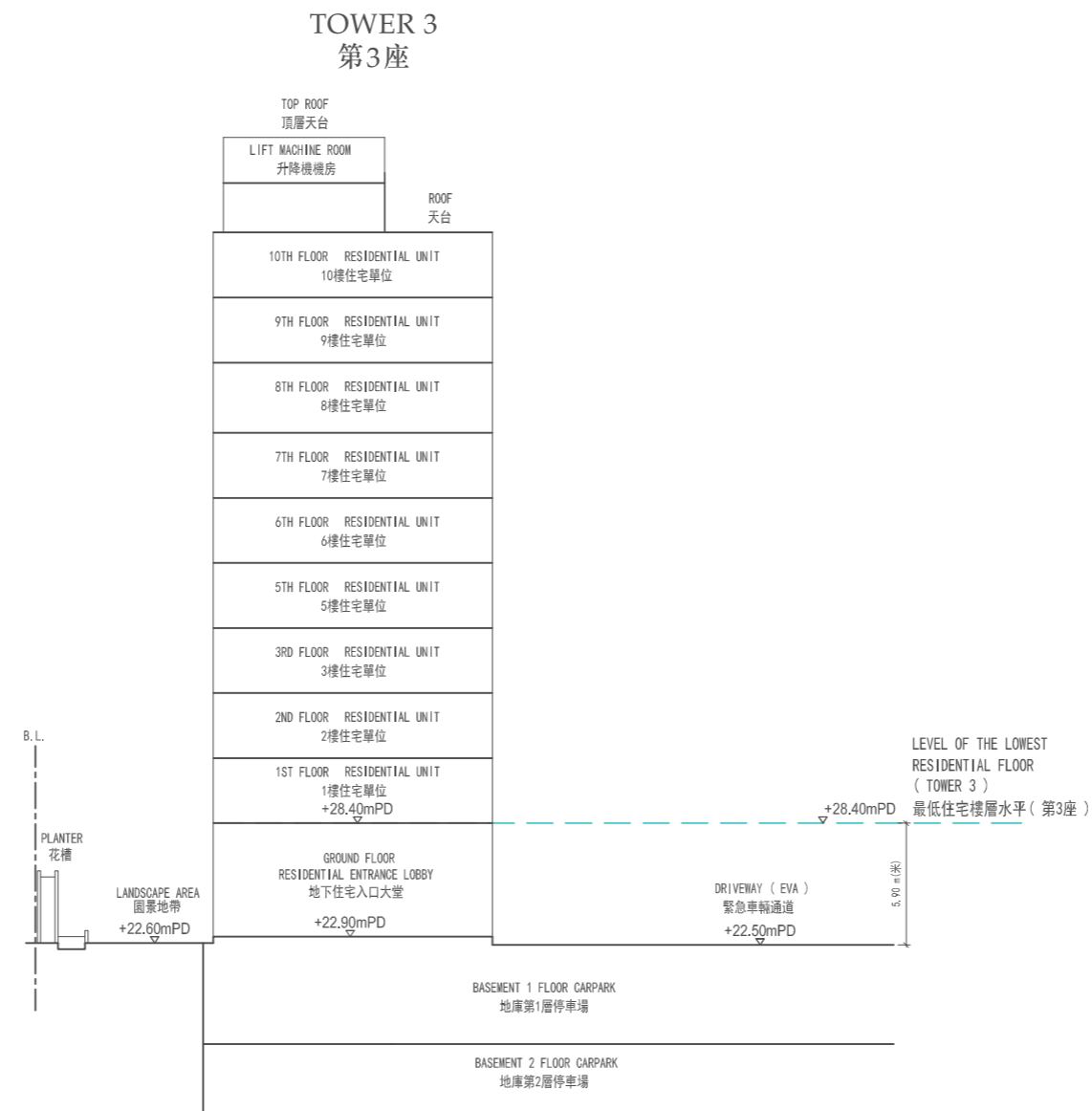
Cross Section Plan C-C 橫截面圖 C-C
