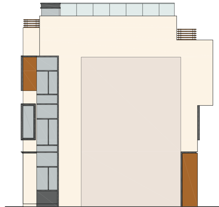
HOUSE C 獨立屋 C
