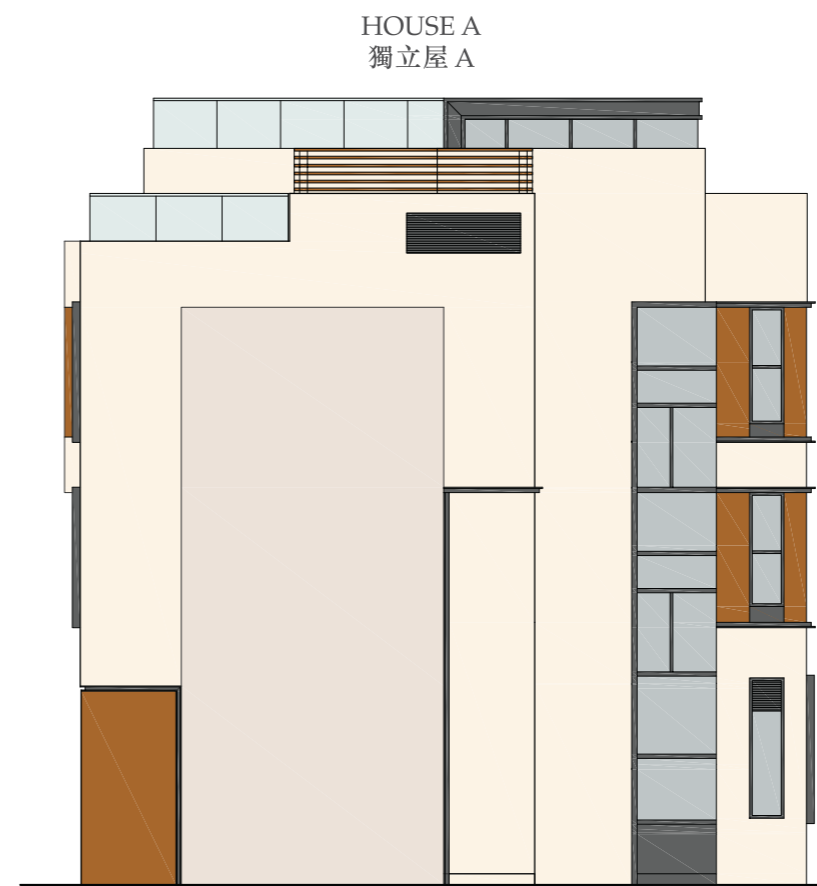
Elevation 8 立面圖 8
