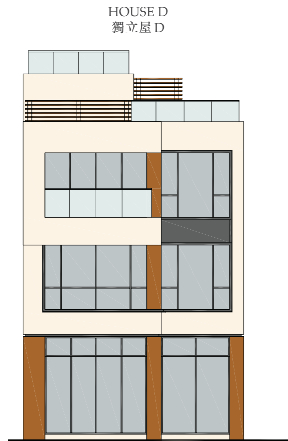
Elevation 17 立面圖 17
