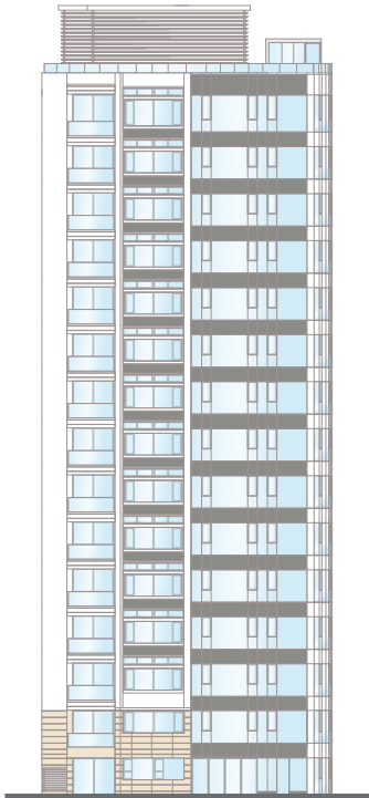
NORTH ELEVATION 北面立面圖
