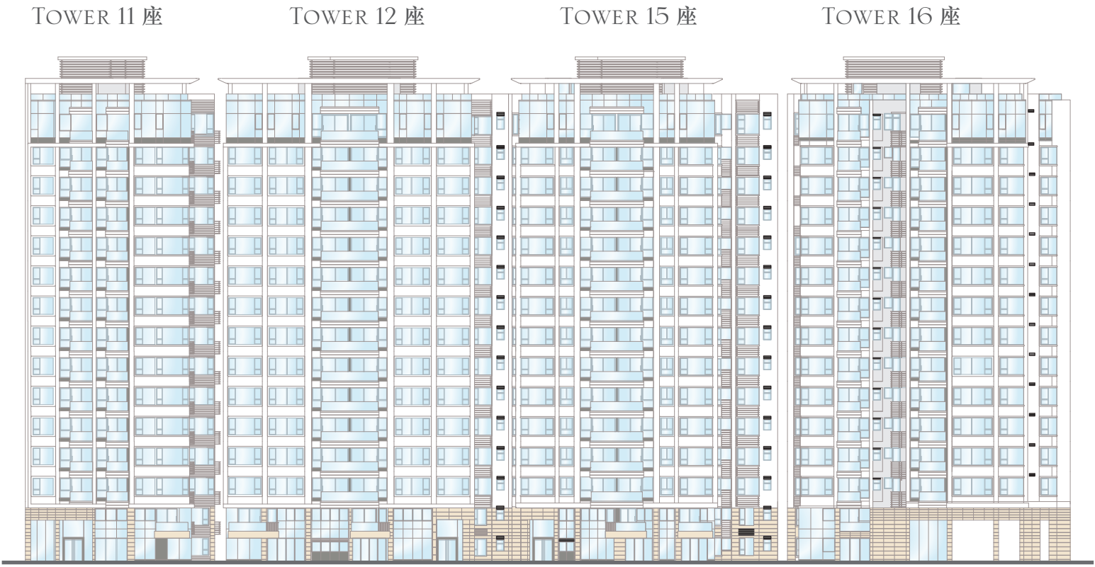
SOUTH ELEVATION 南面立面圖
