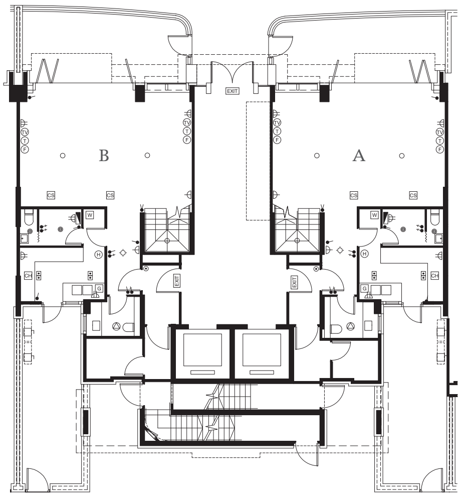
TOWER 6 — UNITS A AND B OF G/F 第六座地下A及B單位
