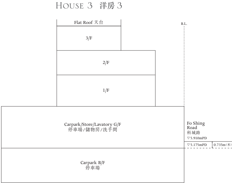
CROSS-SECTION PLAN P 橫截面圖 P
