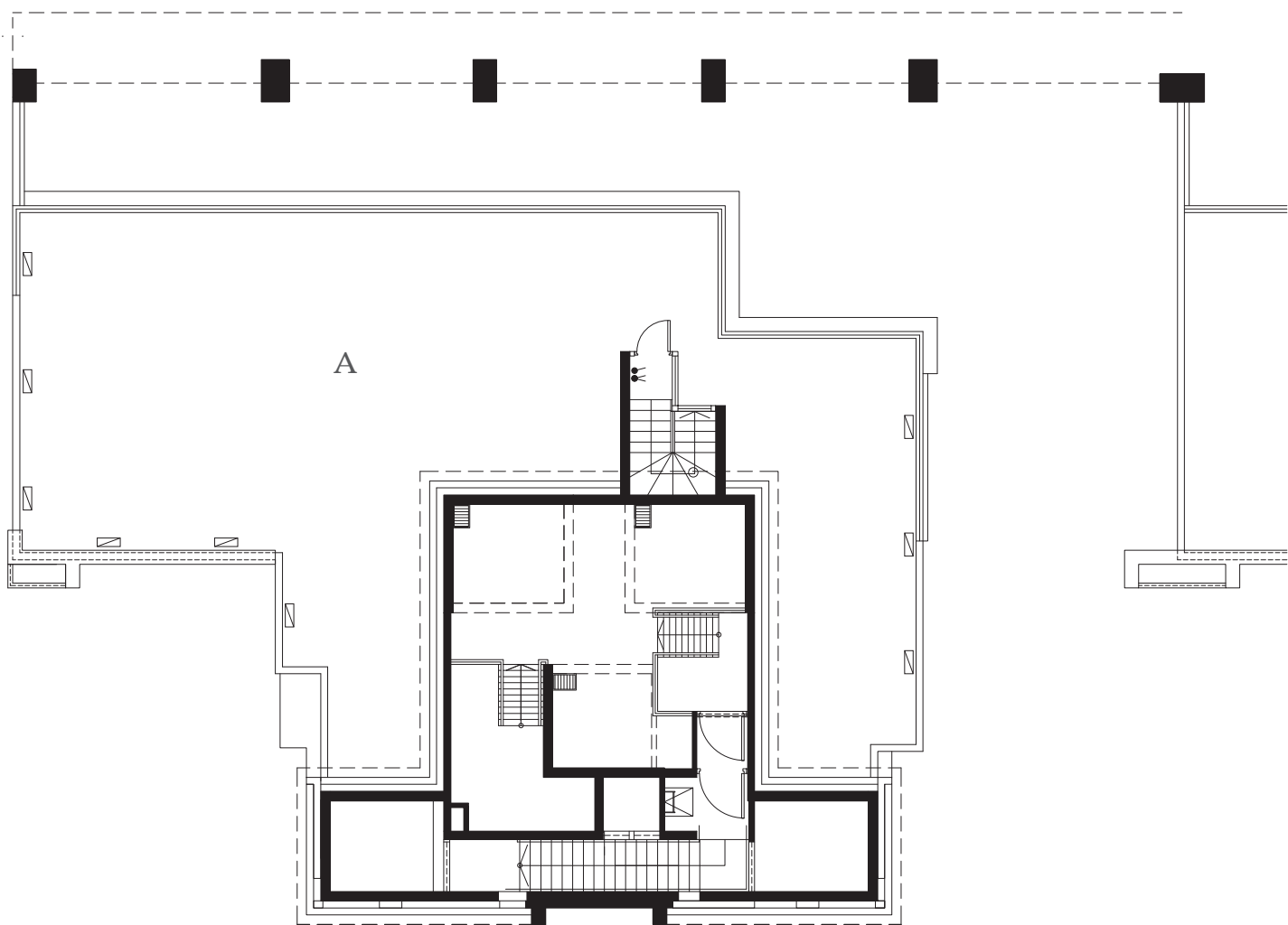
TOWER 5 — UNIT A OF R/F 第五座天台A單位
