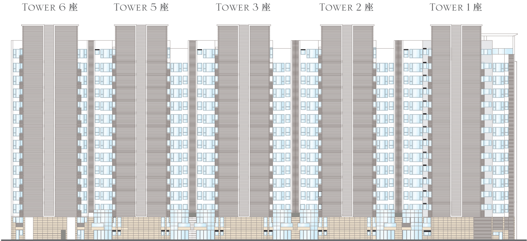
SOUTH WEST ELEVATION 西南面立面圖
