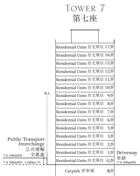
CROSS-SECTION PLAN F 橫截面圖 F
