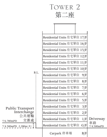
CROSS-SECTION PLAN B 橫截面圖 B
