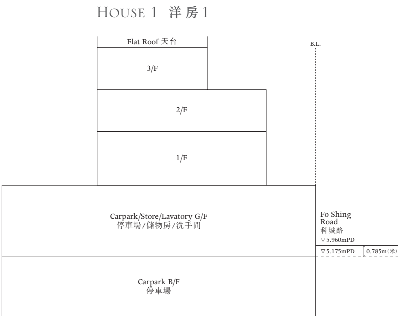
CROSS-SECTION PLAN N 橫截面圖 N
