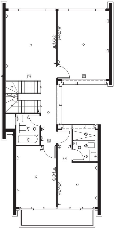
HOUSE 11 — SECOND FLOOR 11號洋房二樓
