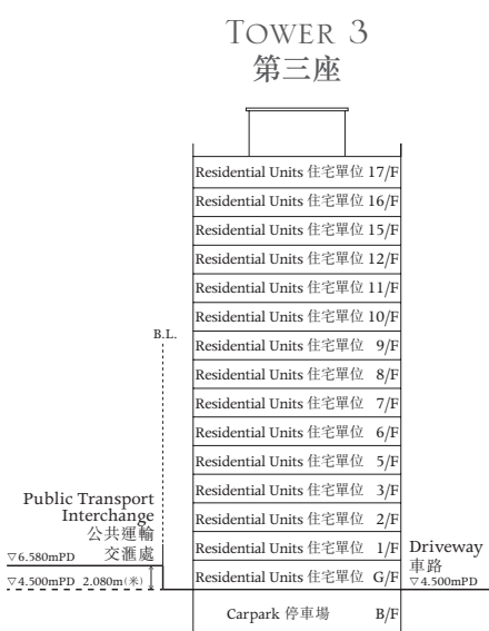
CROSS-SECTION PLAN C 橫截面圖 C
