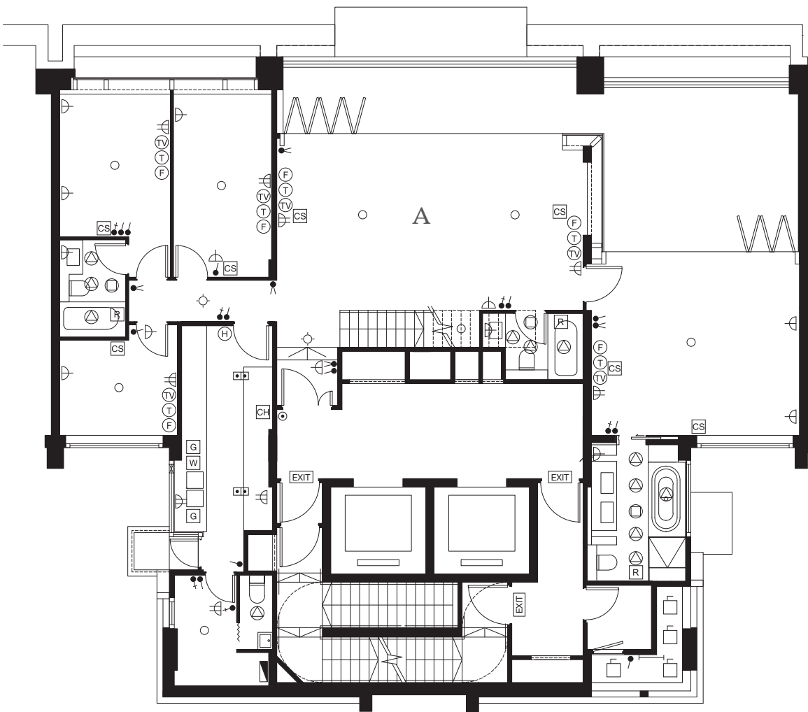
TOWER 6 — UNIT A OF 17/F 第六座十七樓A單位
