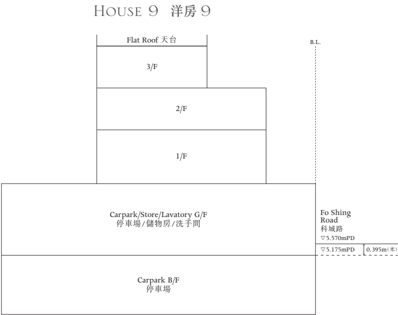
CROSS-SECTION PLAN U 橫截面圖 U
