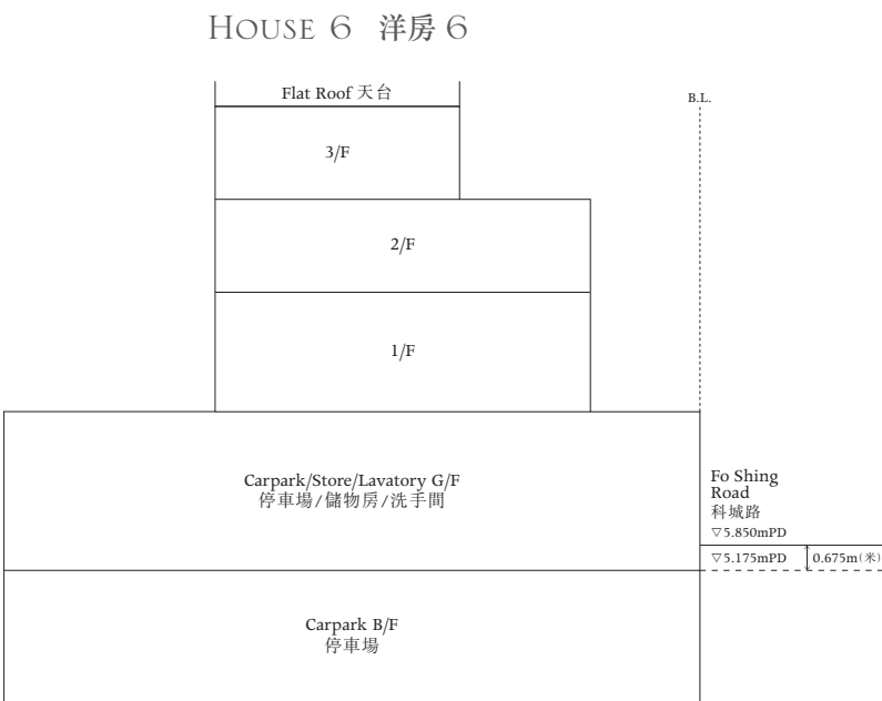
CROSS-SECTION PLAN R 橫截面圖 R
