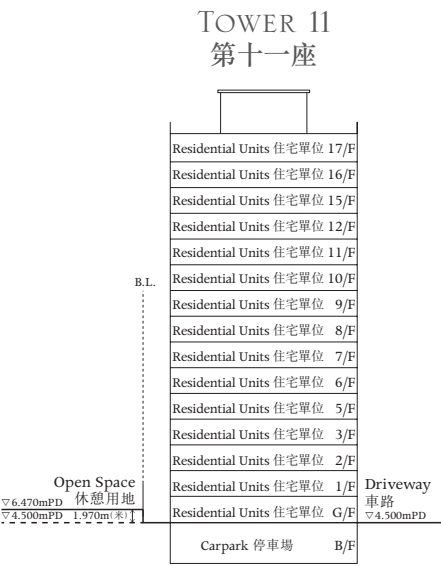
CROSS-SECTION PLAN J 橫截面圖 J
