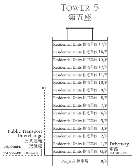
CROSS-SECTION PLAN D 橫截面圖 D
