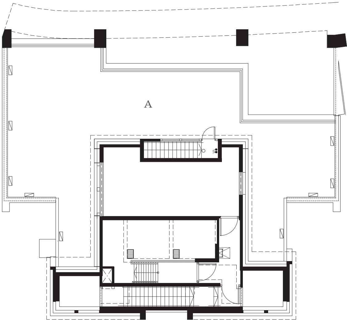
TOWER 8 — UNIT A OF R/F 第八座天台A單位
