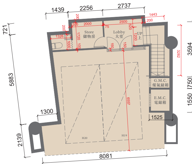
Ground Floor Plan 地下平面圖
