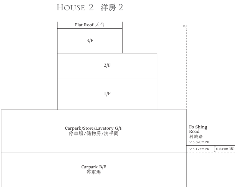
CROSS-SECTION PLAN O 橫截面圖 O
