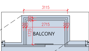
1/F Plan in "as-is" Layout 一樓現狀部分平面圖
