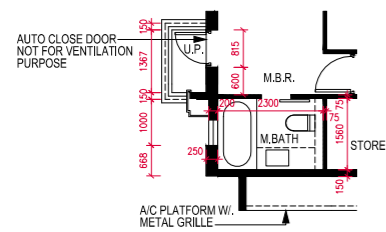
15/F PART PLAN 15樓局部平面圖
