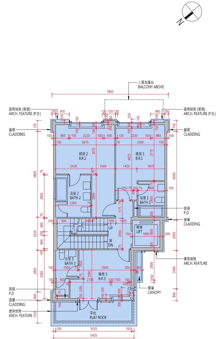
1樓平面圖 1/F Floor Plan
