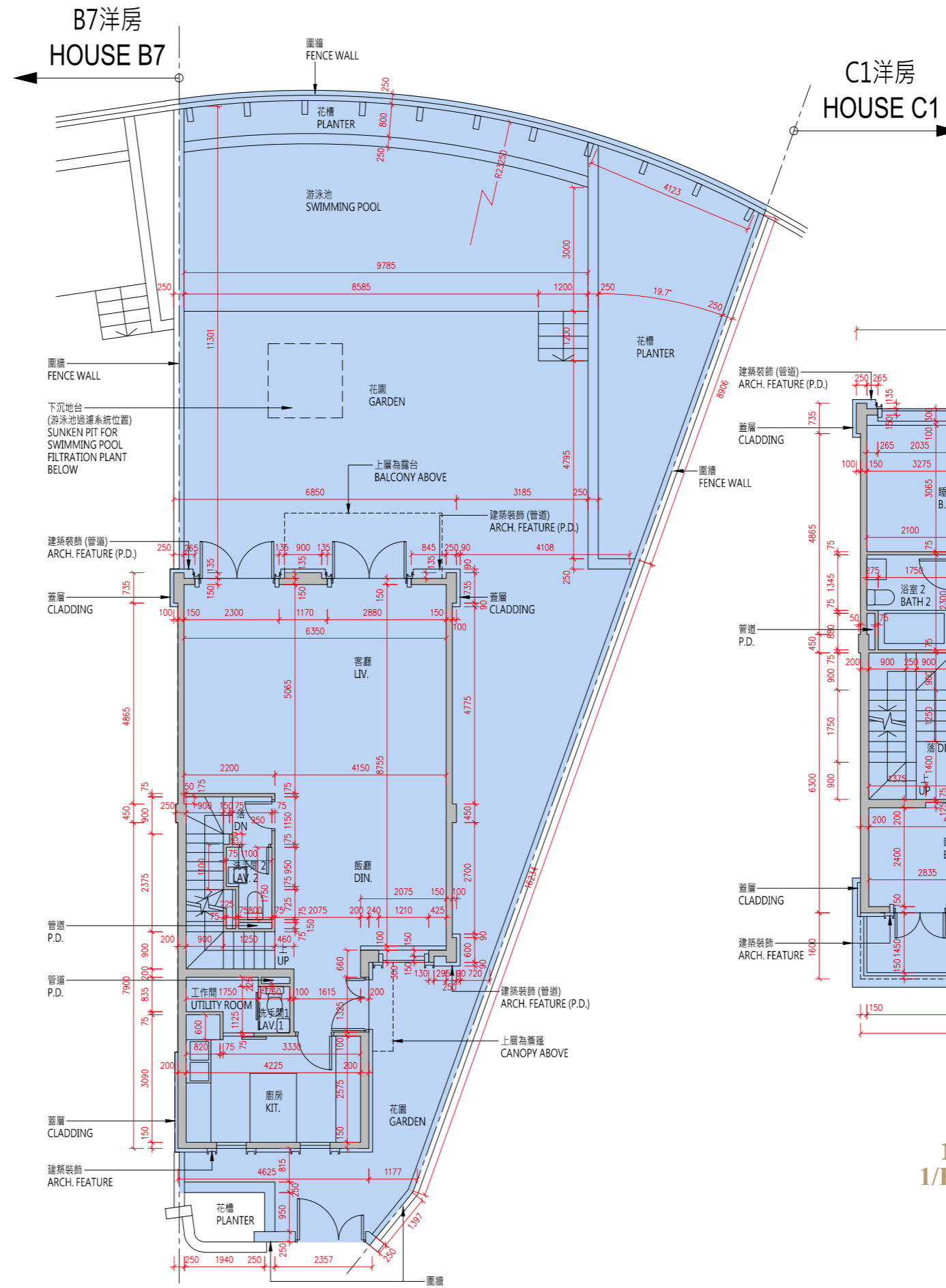
地下平面圖 G/F Floor Plan
