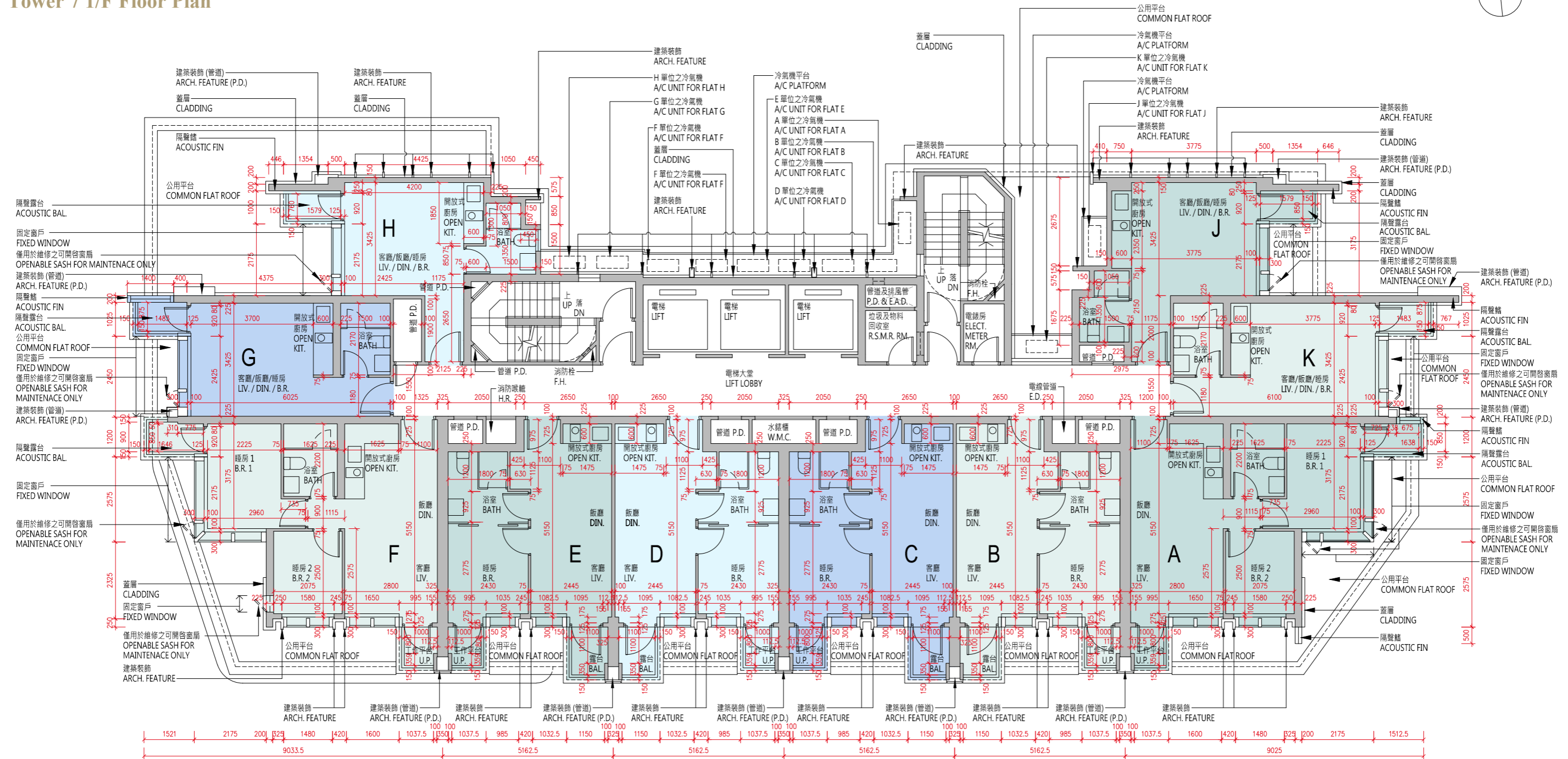
第7座 1樓平面圖 Tower 7 1/F Floor Plan
