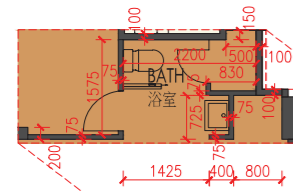
2/F Floor Plan 2樓平面圖
