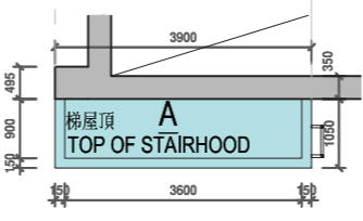
Upper Roof Part Plan 上層天台樓面局部平面圖
