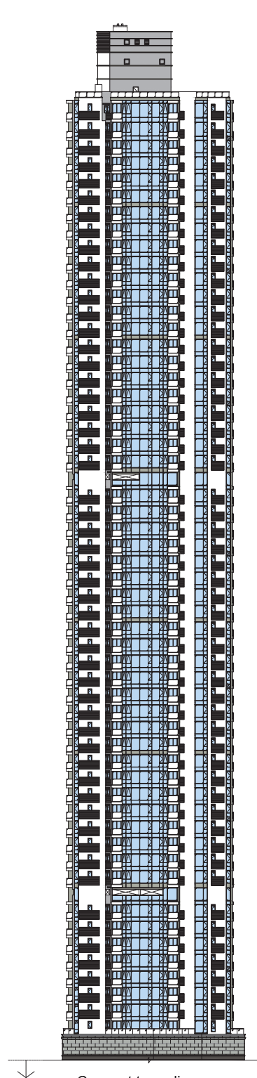
Elevation C2 立面圖 C2
