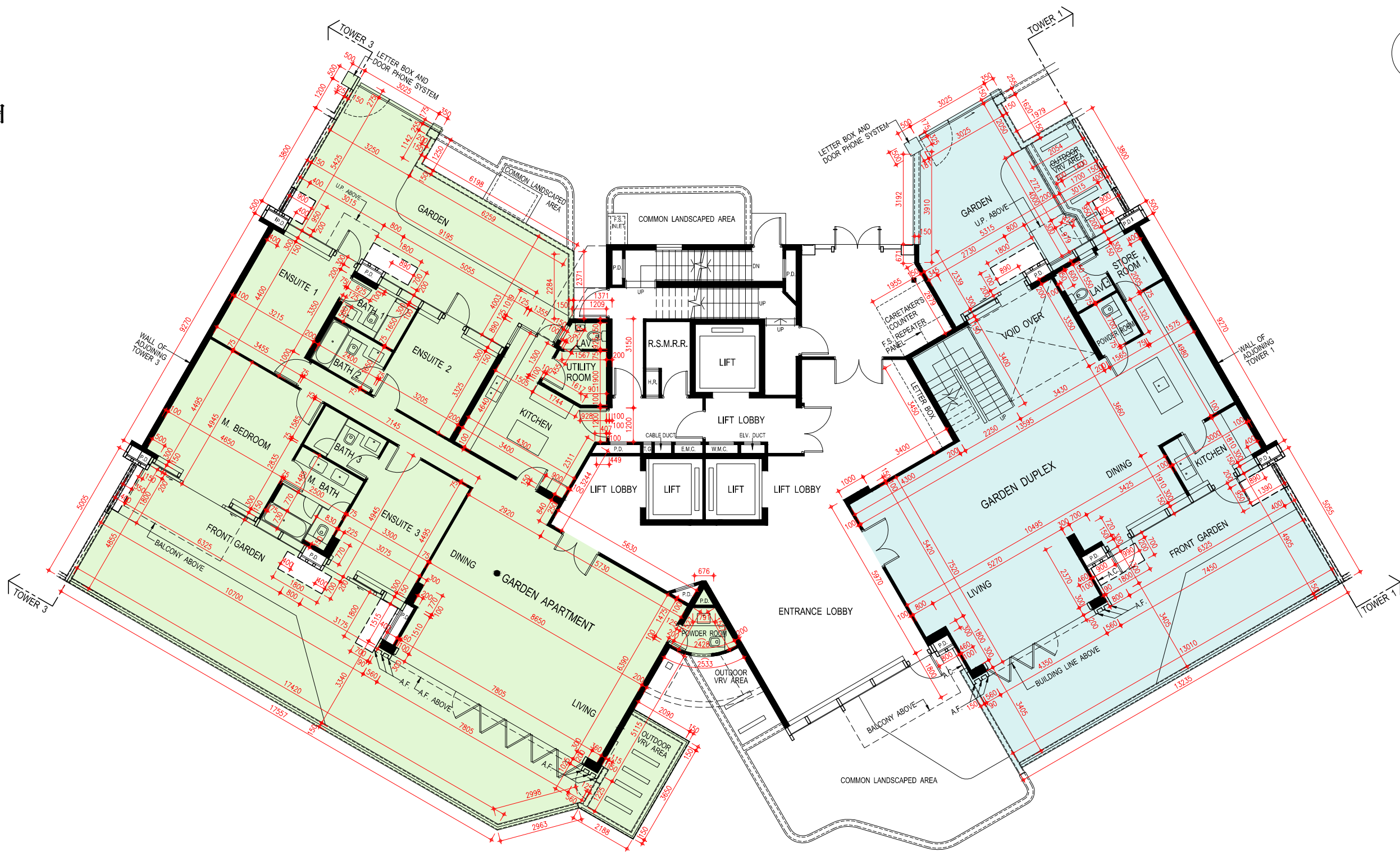
Tower 2 第2座 G/F Plan 地下平面圖
