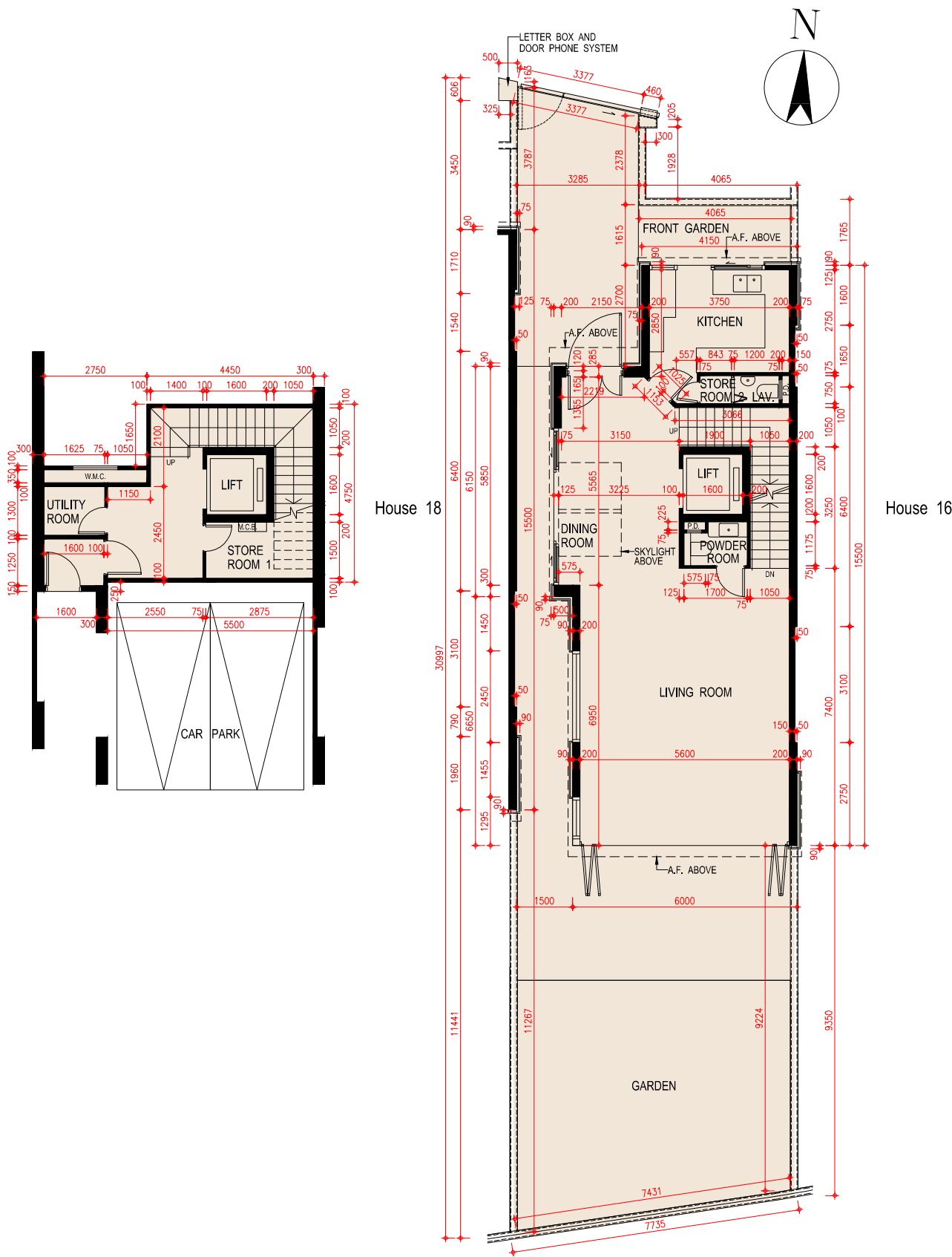
Basement Plan 地庫平面圖
