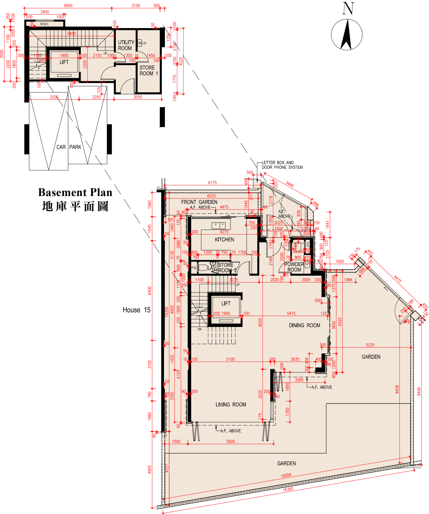
G/F Plan 地下平面圖
