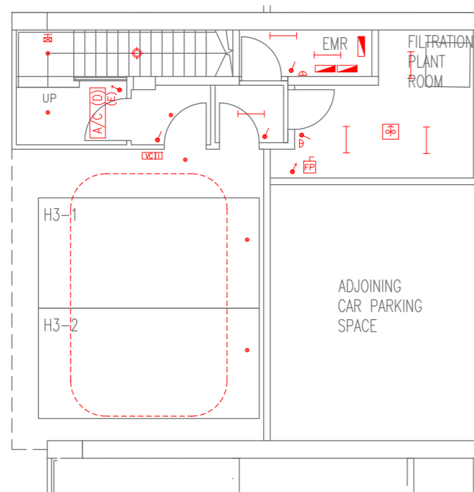
HOUSE CARPARK LEVEL PLAN 獨立屋停車層平面圖
