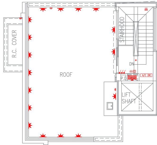
HOUSE ROOF PLAN 獨立屋天台平面圖
