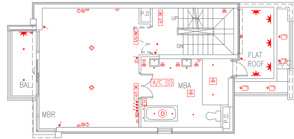
HOUSE LEVEL 3 PLAN 獨立屋第三層平面圖
