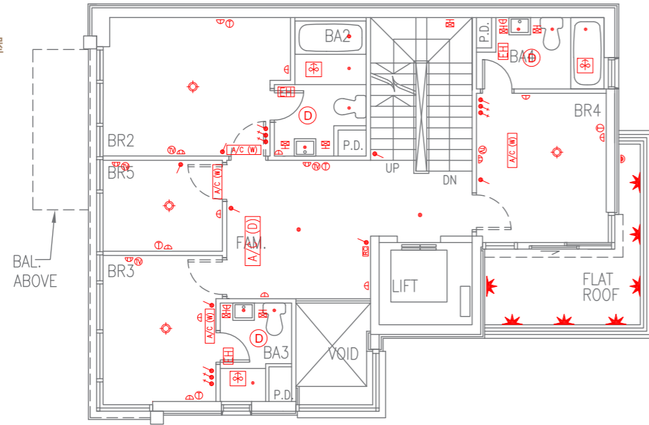
HOUSE LEVEL 2 PLAN 獨立屋第二層平面圖
