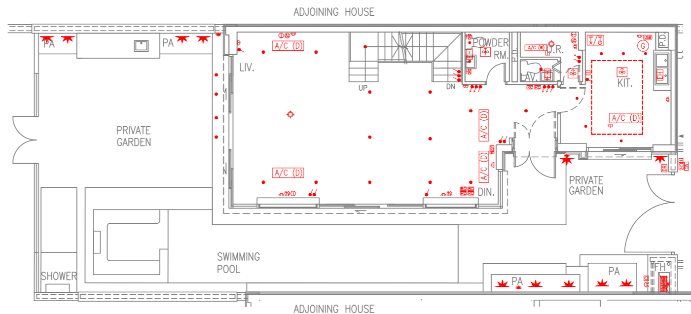
HOUSE LEVEL 1 PLAN 獨立屋第一層平面圖
