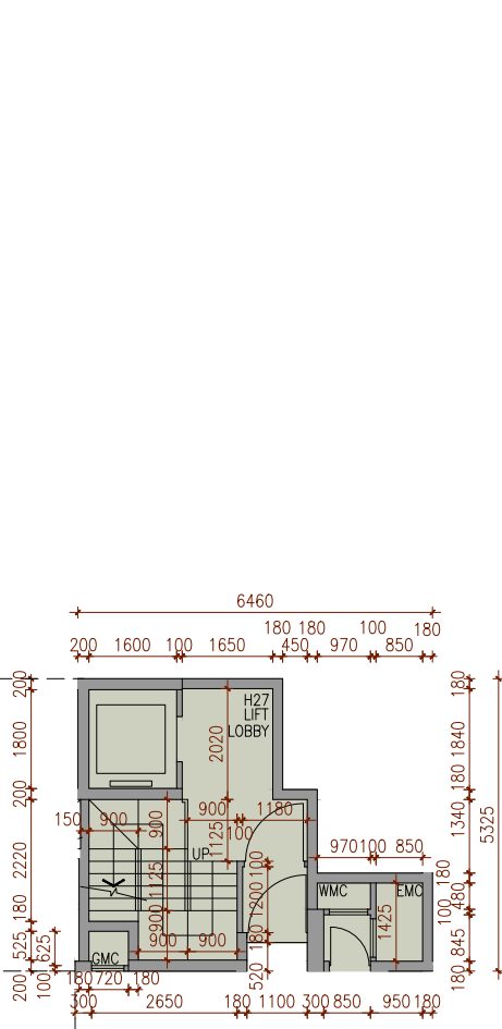
BASEMENT FLOOR PLAN 地庫層平面圖
