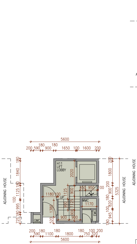
BASEMENT FLOOR PLAN 地庫層平面圖
