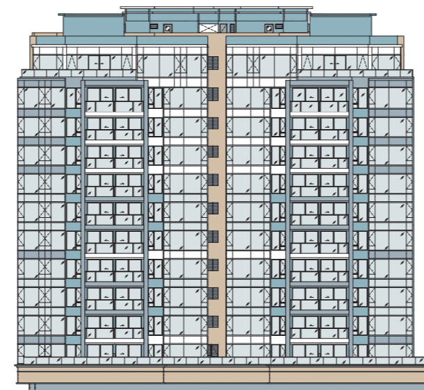
Elevation 4 立面 4
