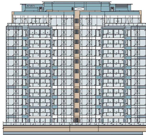
Elevation 2 立面 2
