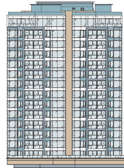
Elevation 4 立面 4
