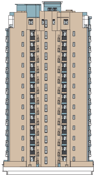
Elevation 3 立面 3
