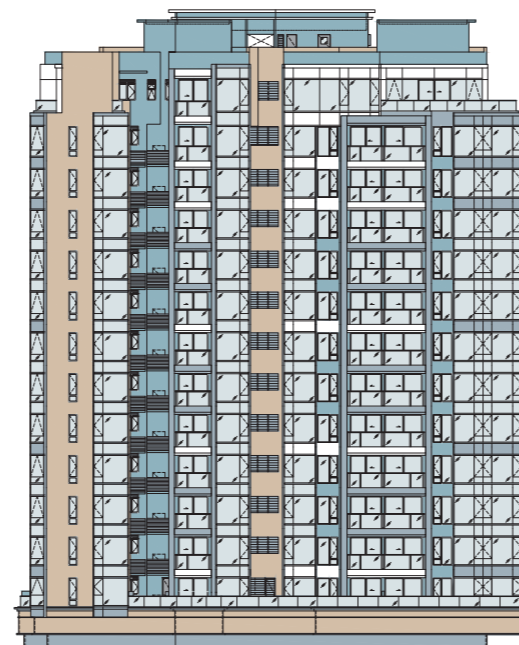
Elevation 4 立面 4
