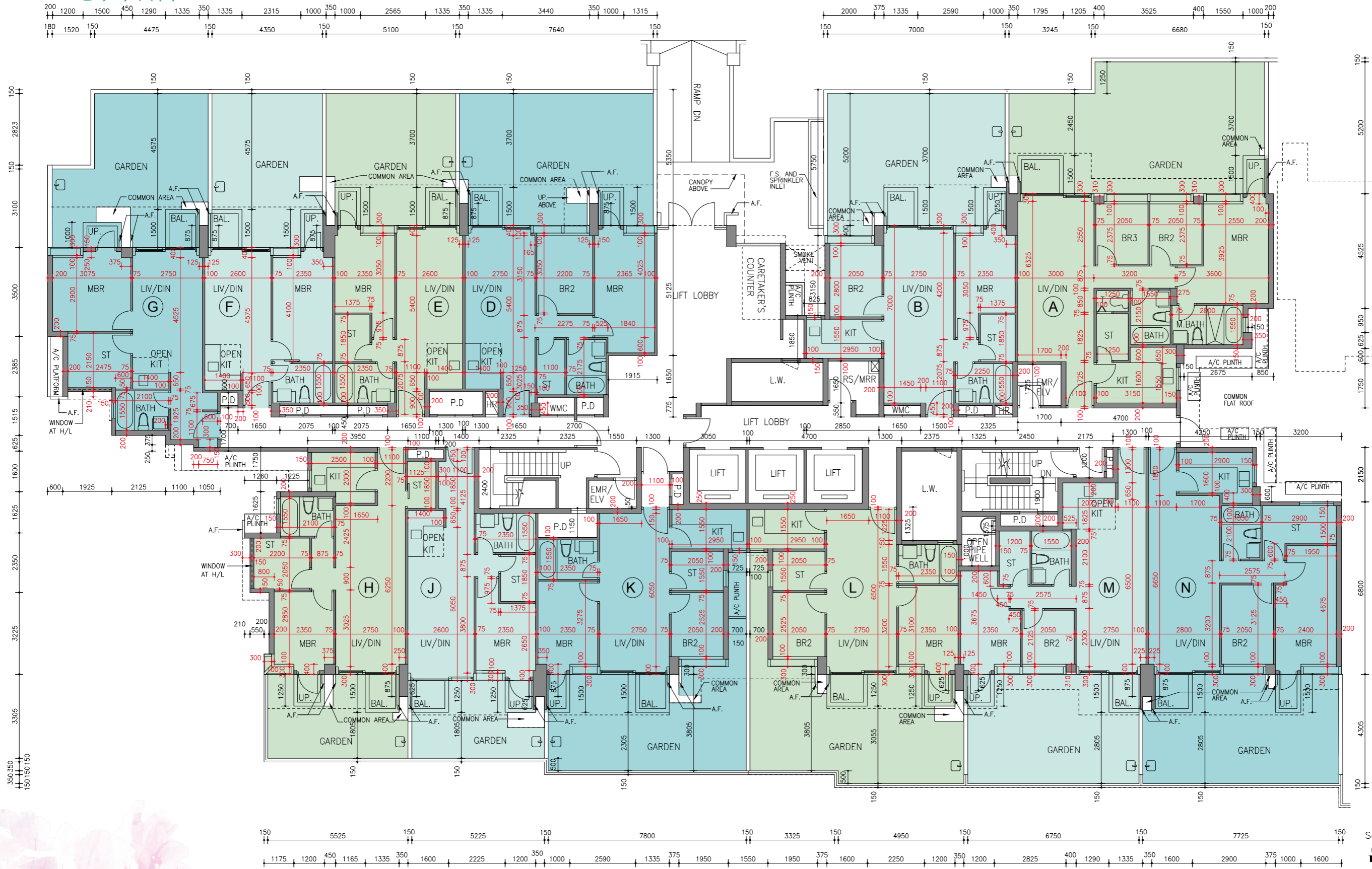
TOWER 2 第二座 GROUND FLOOR PLAN 地下平面圖
