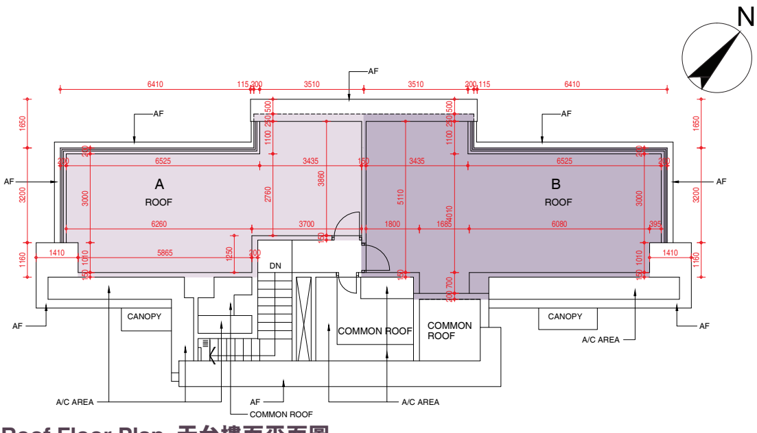
Roof Floor Plan 天台樓面平面圖
