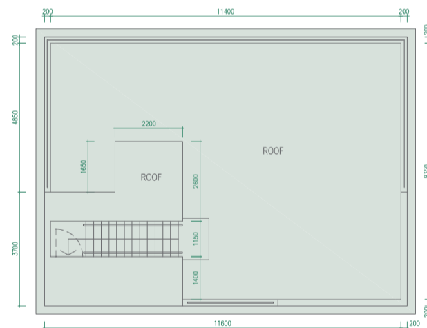
Floor Plan R/F 天台平面圖
