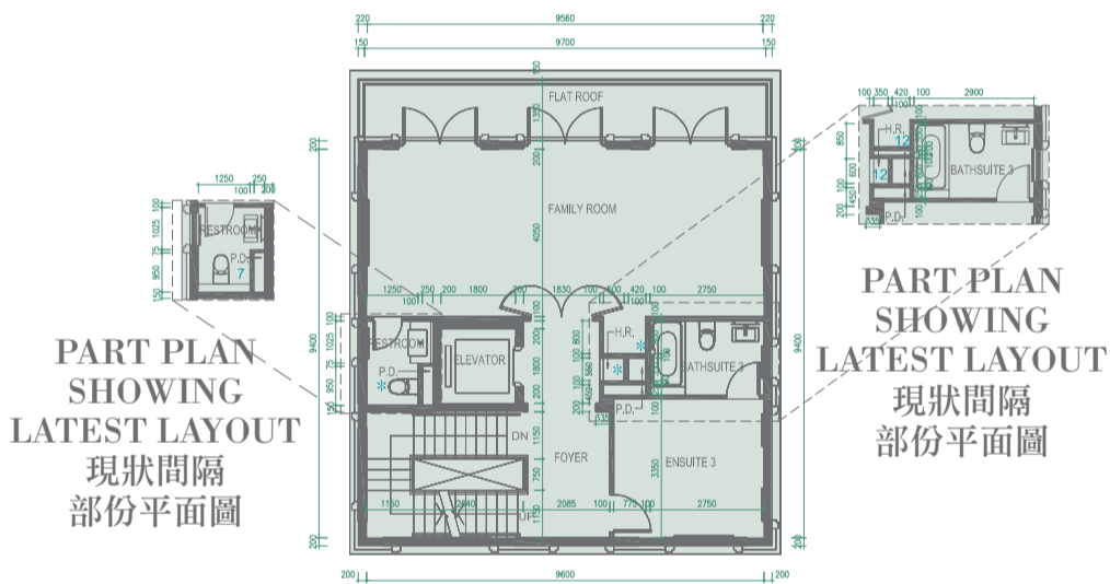
Floor Plan 3/F 三樓平面圖
