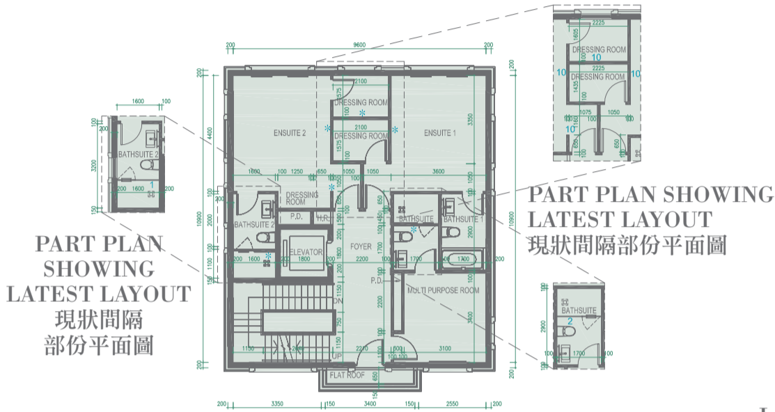
Floor Plan 1/F 一樓平面圖
