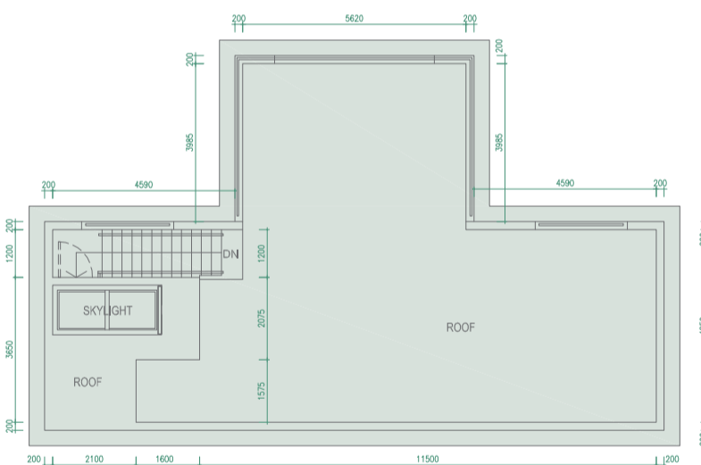
Floor Plan R/F 天台平面圖
