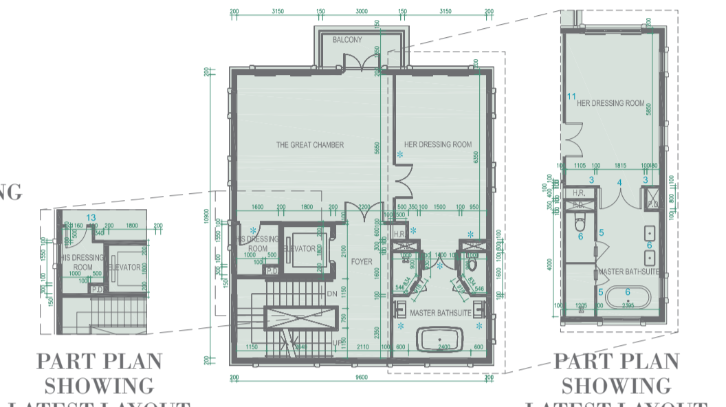
Floor Plan 2/F 二樓平面圖
