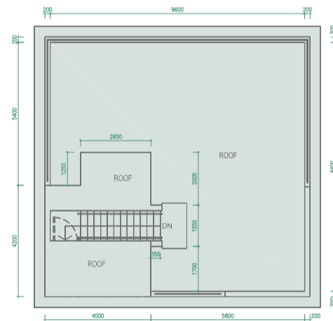
Floor Plan R/F 屋頂平面圖
