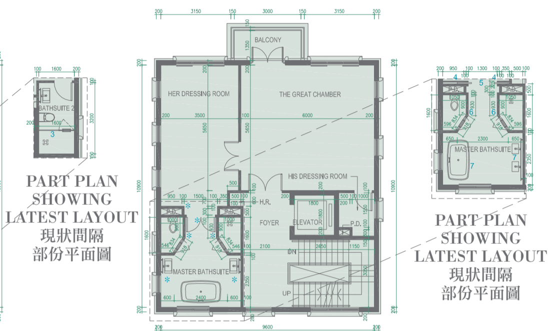
Floor Plan 2/F 二樓平面圖
